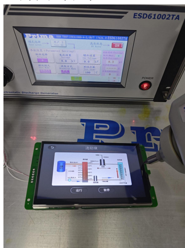
图 5-2 ESD 测试图
