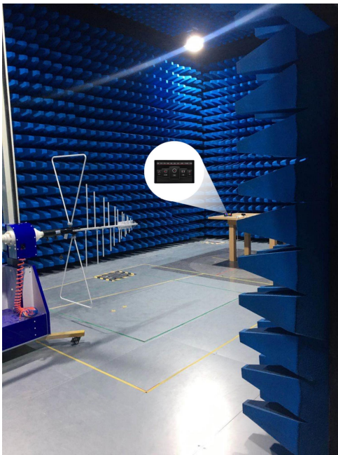
图 5-5 辐射测试图
