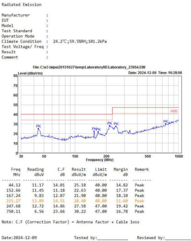
图 5-6 辐射测试水平方向
